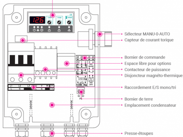
TZ1 Module de commande embrochable
